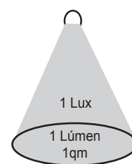
Luminancia L
