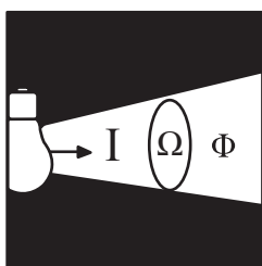
Flujo Luminoso
